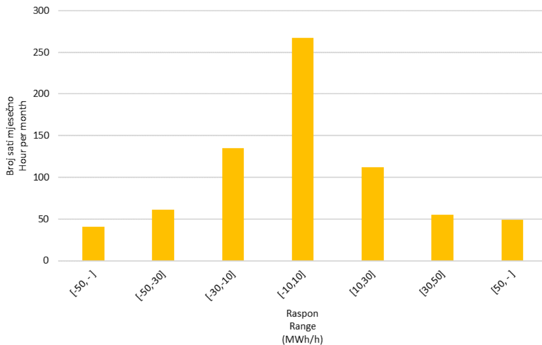
Slika 10 Statistička raspodjela satnih promjena proizvodnje VE u rujnu 2020. godine Figure 10 Statistical distribution of WPP hourly output variations in September 2020
