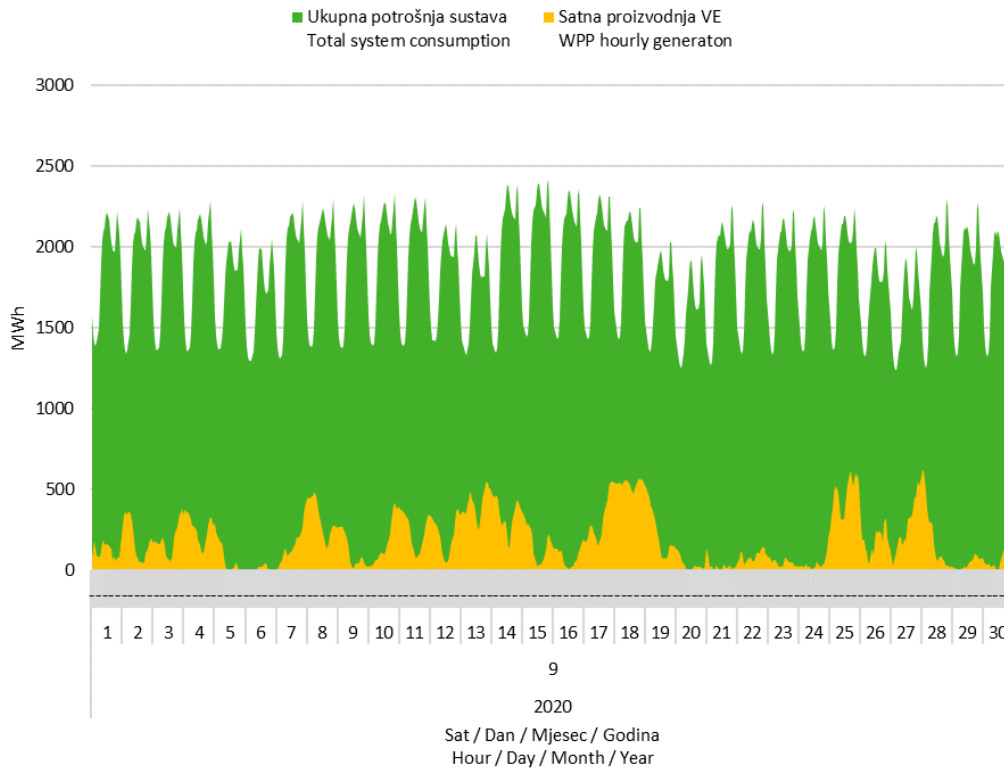
Slika 7 Usporedba satnog dijagrama opterećenja sustava i proizvodnje vjetroelektrana u rujnu 2020. godine
