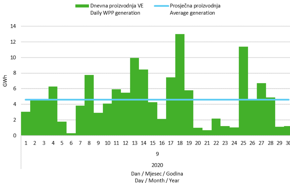
Slika 5 Dnevna proizvodnja svih vjetroelektrana u rujnu 2020. godine Figure 5 Daily generation of all wind power plants in September 2020
