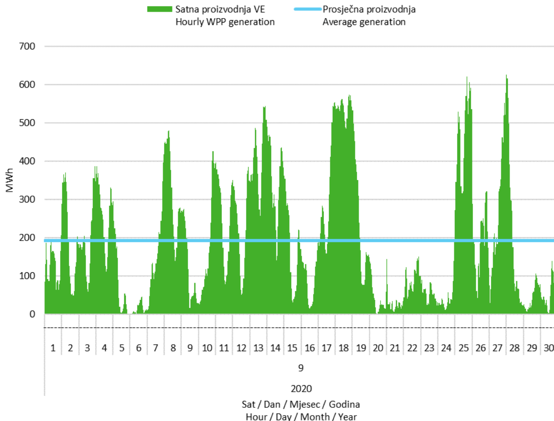
Slika 2 Satna proizvodnja svih vjetroelektrana u rujnu 2020. godine Figure 2 Hourly generation of all wind power plants in September 2020
