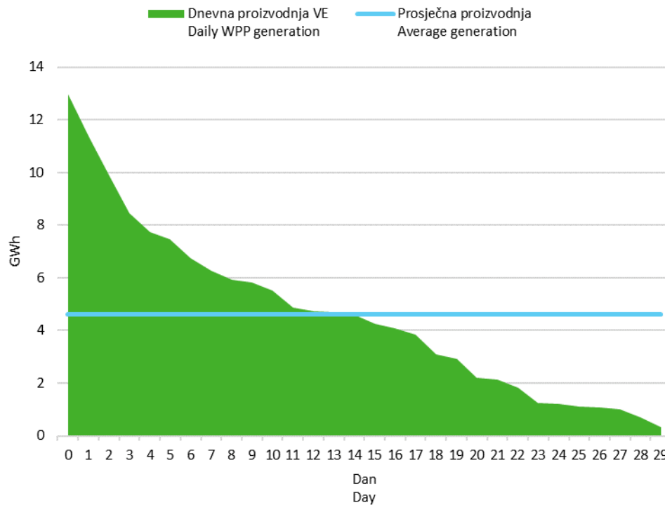
Slika 6 Krivulja trajanja dnevne proizvodnje vjetroelektrana u rujnu 2020. godine
