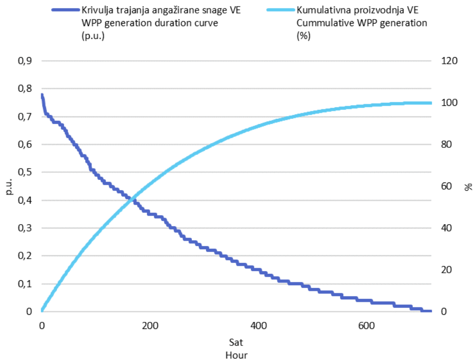
Slika 3 Krivulja trajanja angažirane snage svih VE i kumulativna proizvodnja VE u rujnu 2020. godine u jediničnim vrijednostima
