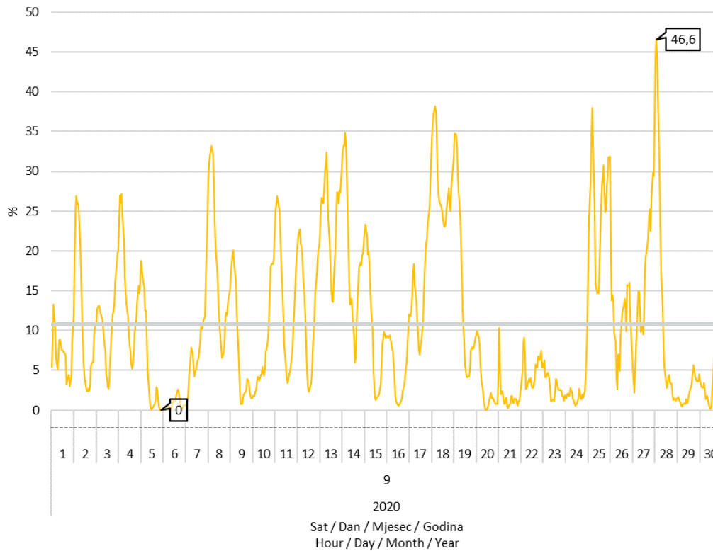
Slika 8 Udio proizvodnje vjetroelektrana u pokrivanju satnog opterećenja elektroenergetskog sustava u rujnu 2020. godine
