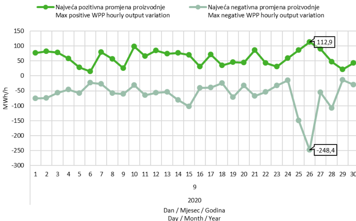
Slika 9 Maksimalna pozitivna i maksimalna negativna promjena satne proizvodnje VE u rujnu 2020. godine
